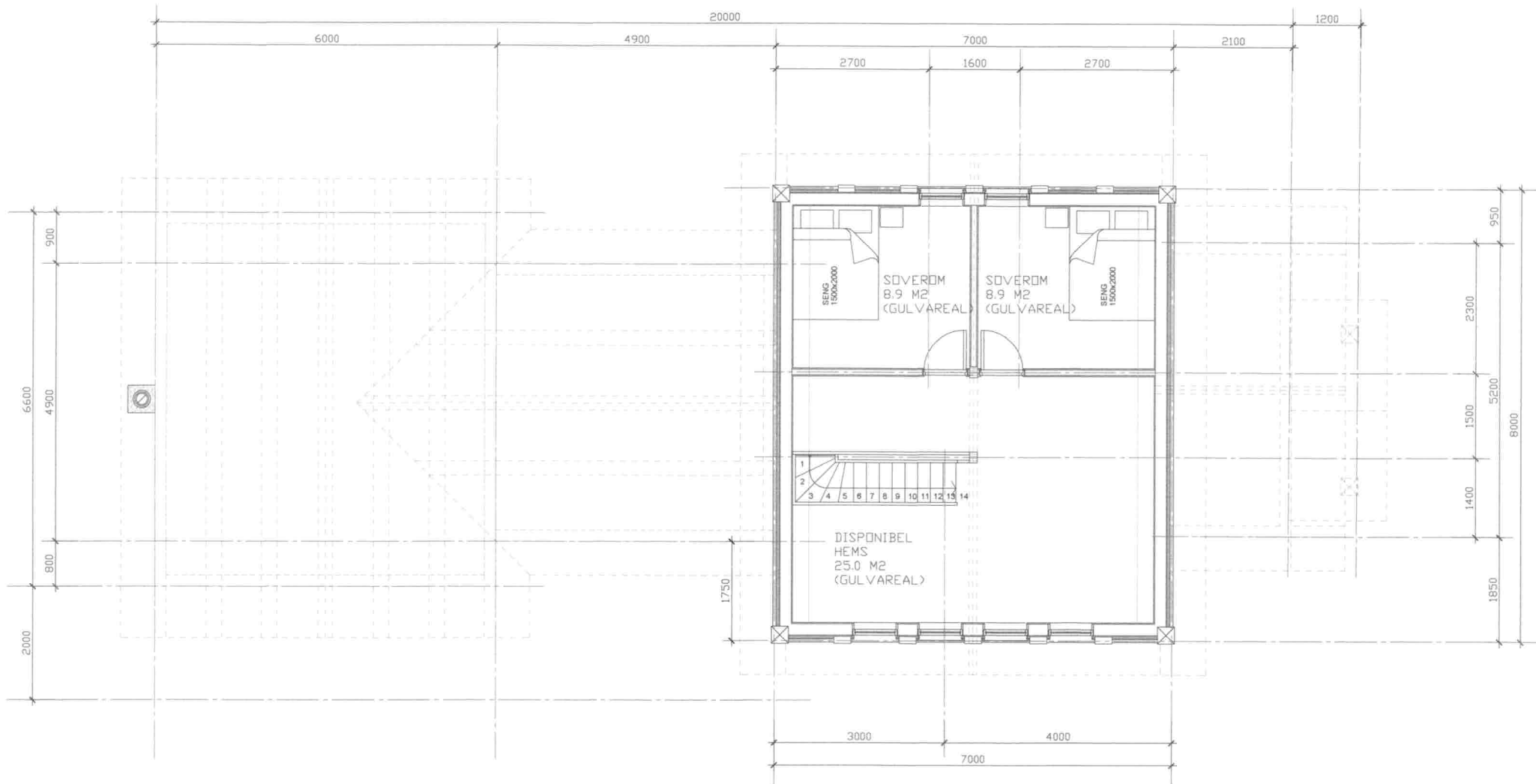
PLAN HEMSETASJE 1:100 BRUKSAREAL: 42.5 M 2
